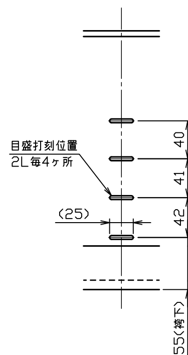
目盛詳細図
