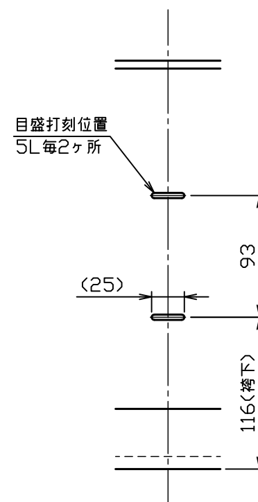
目盛詳細図
