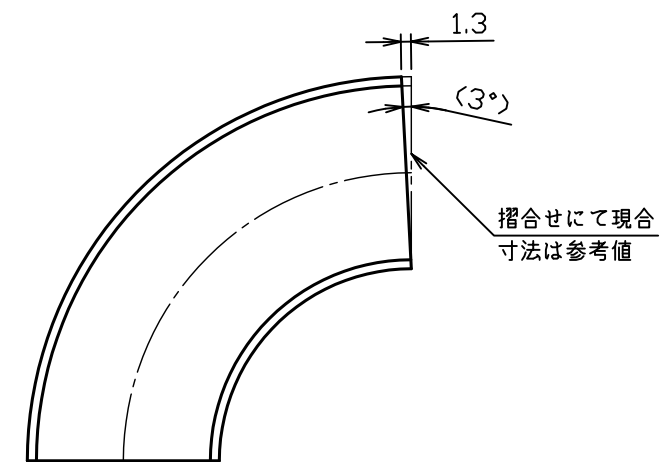
エルボ摺合せ参考図 S = 1 : 1
