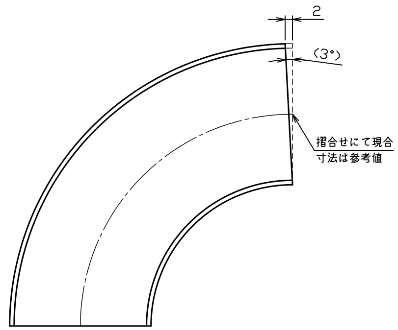
エルボ摺合せ参考図 S = 1 : 1
