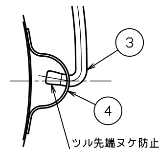
△△ C部詳細図 S = 1 : 2
