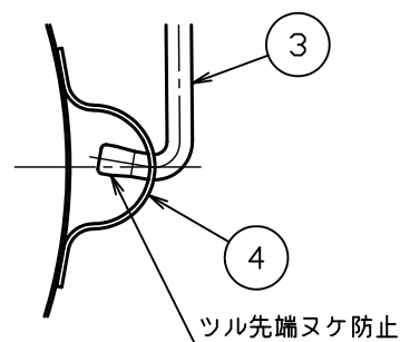
A A部詳細図 S = 1 : 2
