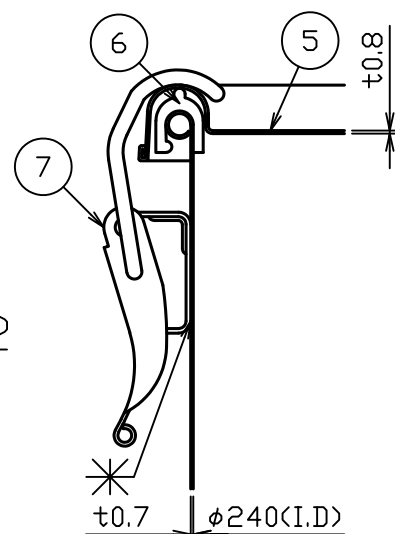
B部詳細図 S = 1 : 2
