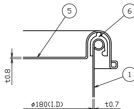
C部詳細図 S = 1 : 1
