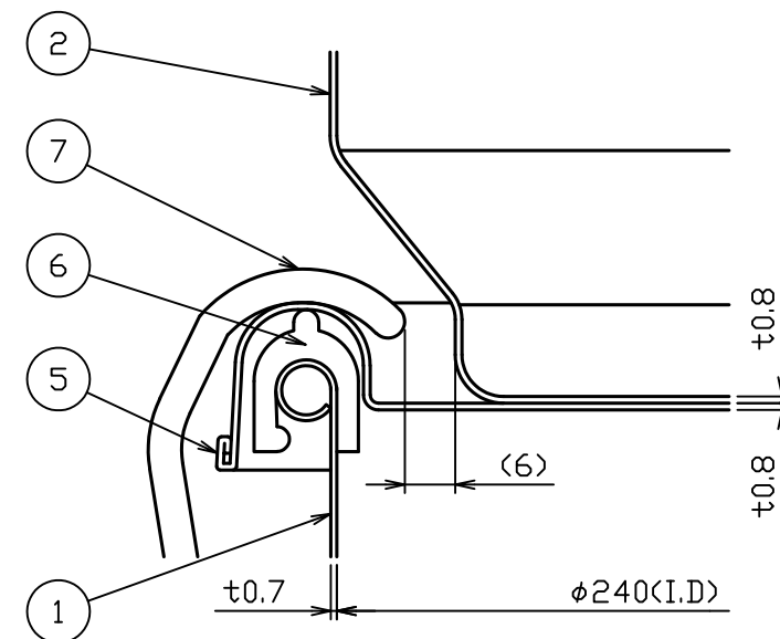
積み重ね詳細図 S = 1 : 1
