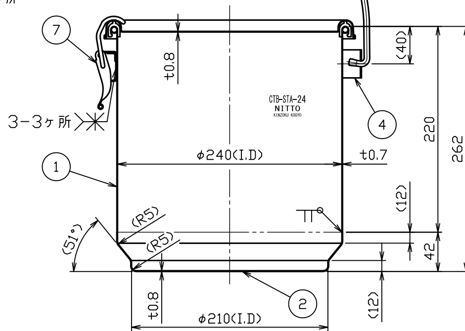
A-A断面図
