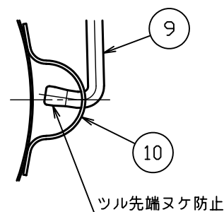
△ C 部詳細図 S = 1 : 2
