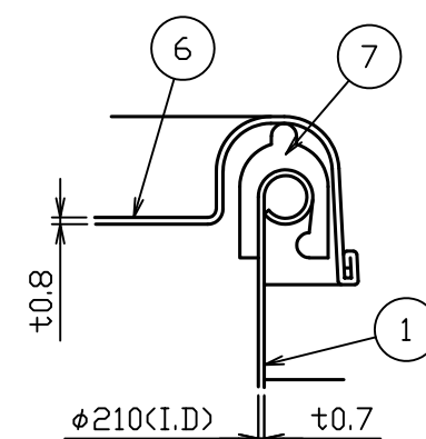
B部詳細図 S = 1 : 1
