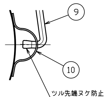
△ C部詳細図 S = 1 : 2
