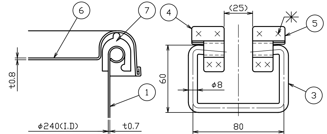
B部詳細図 S = 1 : 1 把手部詳細図 S = 1 : 2
