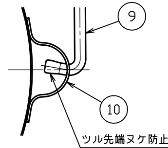
△ C部詳細図 S = 1 : 2
