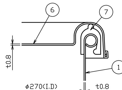
B部詳細図 S = 1 : 1
