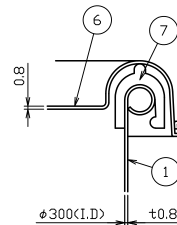
B部詳細図 S = 1 : 1
