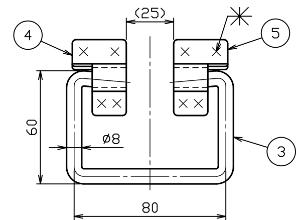
把手部詳細図 S = 1 : 2
