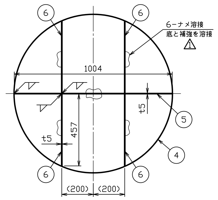
D矢視図
