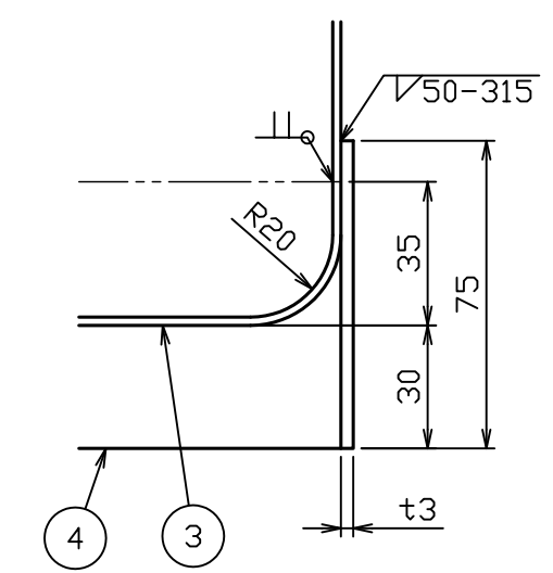
C部詳細図 S=1:2
