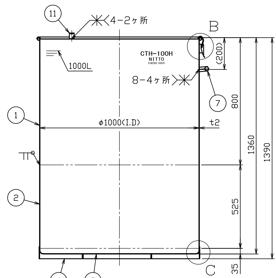
A-A断面図
