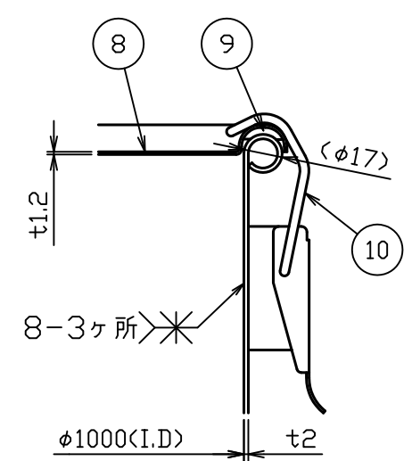
△B部詳細図 S=1:3
