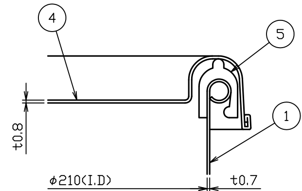
A部詳細図 S = 1 : 1
