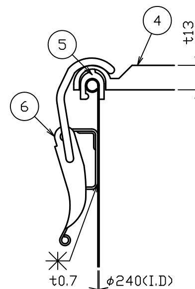
A部詳細図 S = 1 : 2
