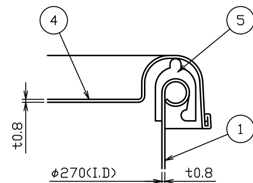
A部詳細図 S = 1 : 1
