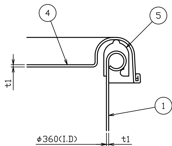
B部詳細図 S = 1 : 1
