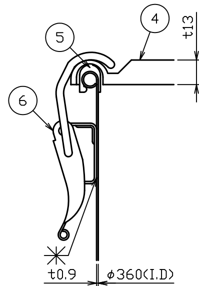
A部詳細図 S = 1 : 2
