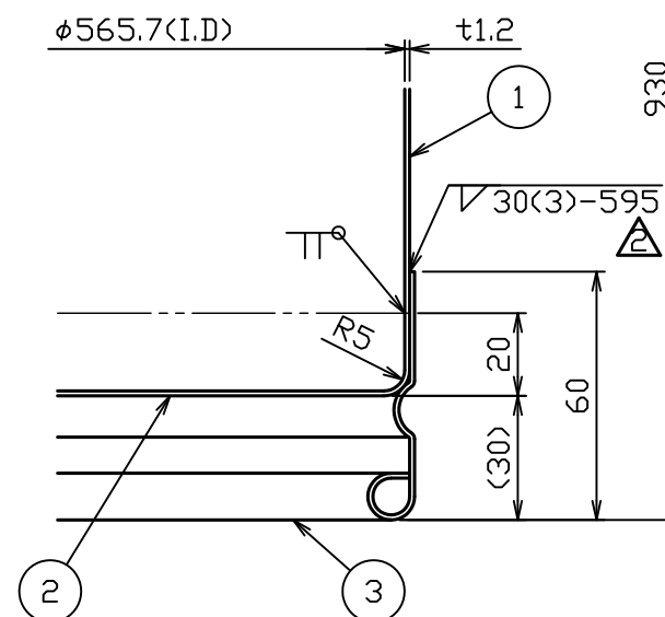
C部詳細図 S = 1 : 2
