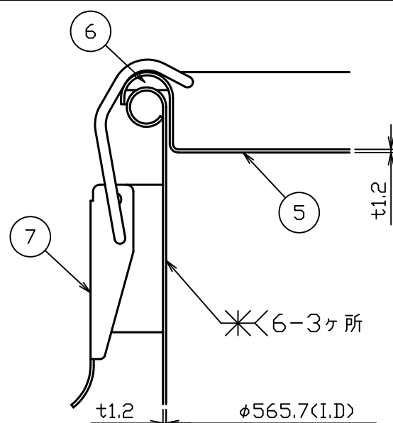
B部詳細図 S = 1 : 2
