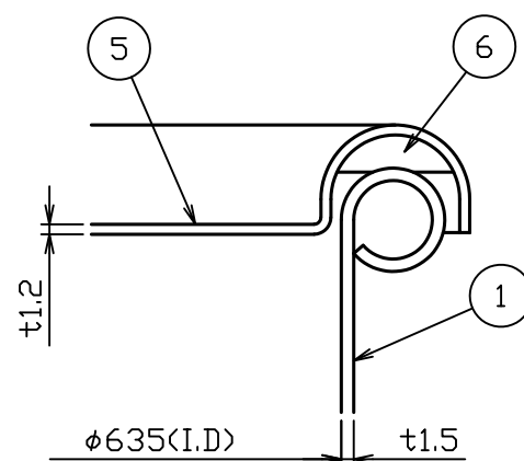
A部詳細図 S = 1 : 1
