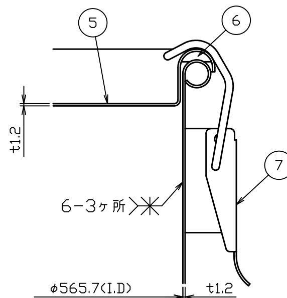
B部詳細図 S = 1 : 2
