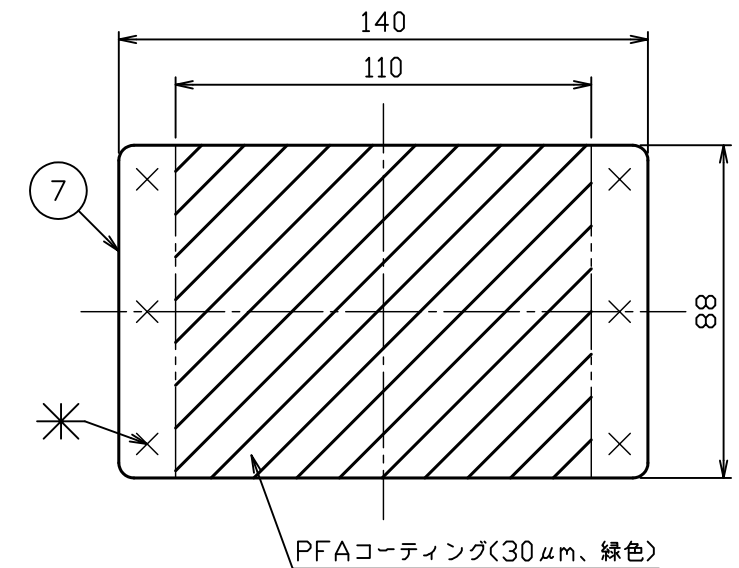
シール座板詳細図 S = 1 : 2
