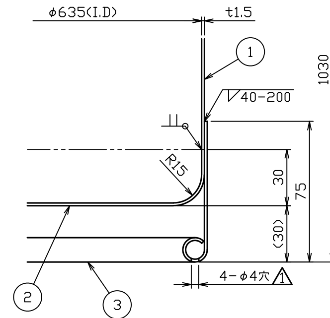
B部詳細図 S = 1 : 2
