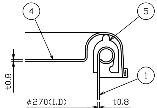
A部詳細図 S = 1 : 1
