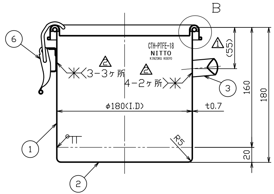
A-A断面図
