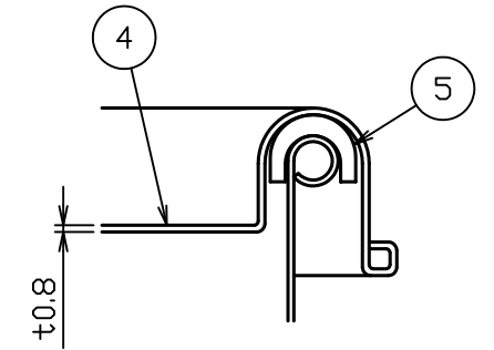
B部詳細図 S = 1 : 1
