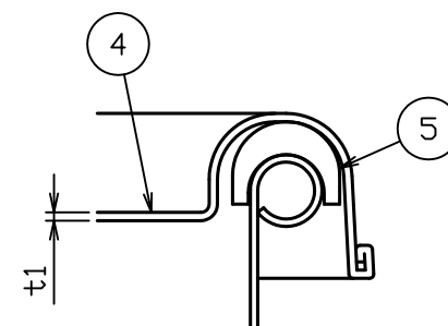
B部詳細図 S = 1 : 1
