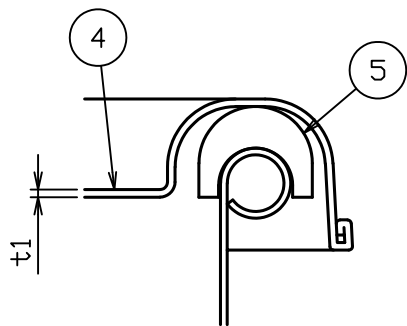
B部詳細図 S = 1 : 1
