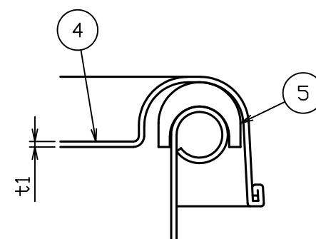
B部詳細図 S = 1 : 1
