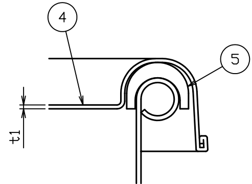
B部詳細図 S = 1 : 1
