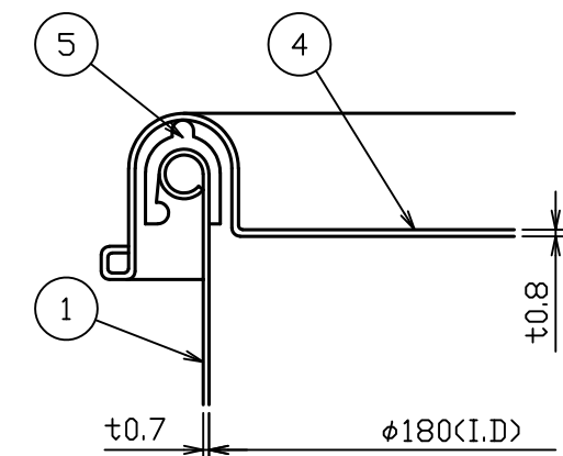
A部詳細図 S = 1 : 1
