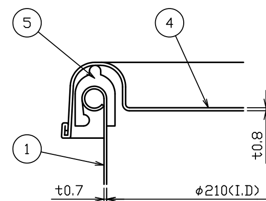
A部詳細図 S = 1 : 1
