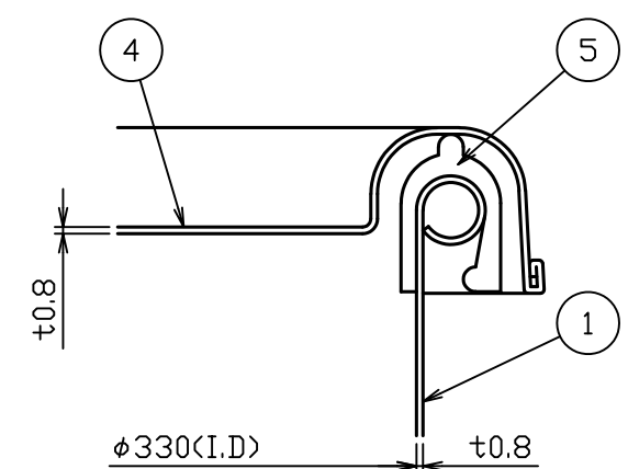
A部詳細図 S = 1 : 1
