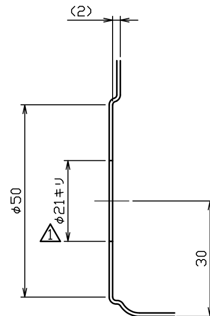
エンボス加工詳細図 S = 1 : 1
