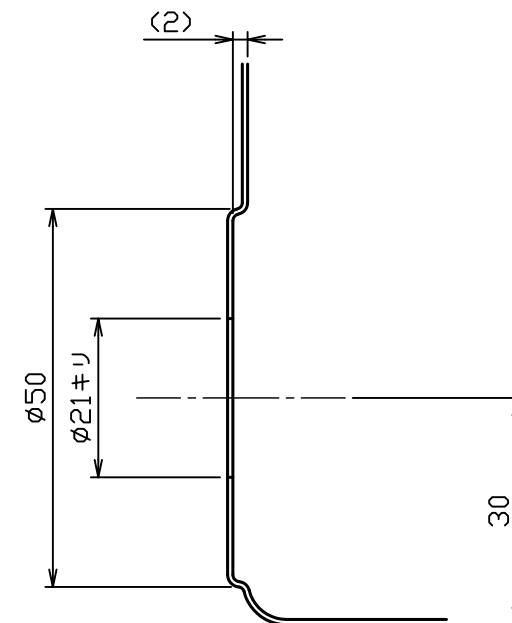
エンボス加工詳細図 S = 1 : 1
