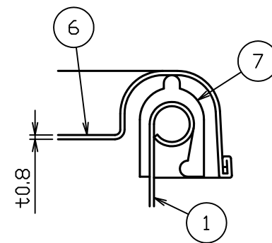
A部詳細図 S = 1 : 1
