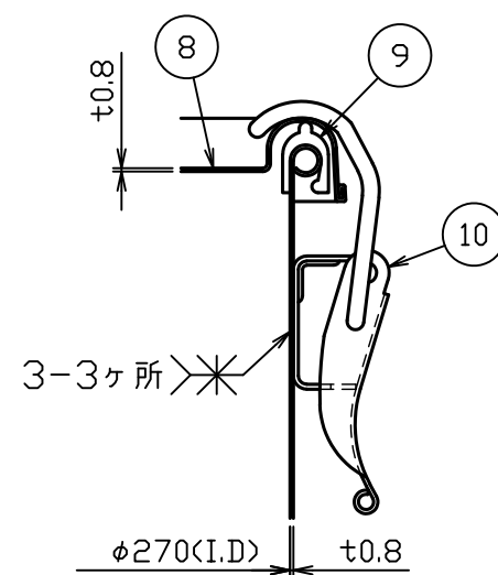
A 部詳細図 S = 1 : 2
