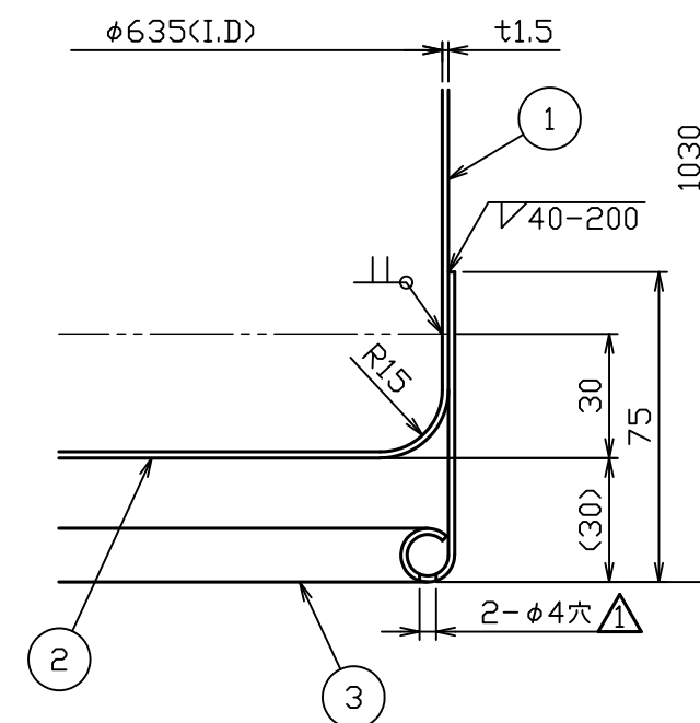
B部詳細図 S = 1 : 2
