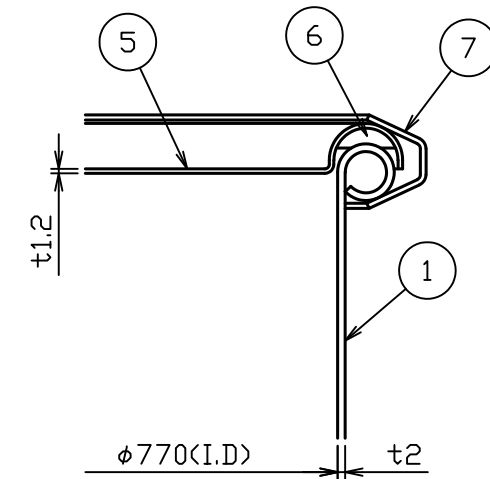
A部詳細図 S = 1 : 2
