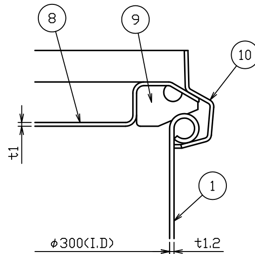
B部詳細図 S = 1 : 1
