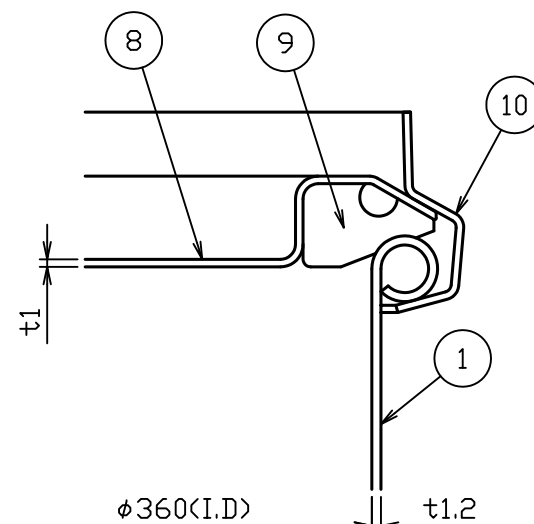
B部詳細図 S = 1 : 1
