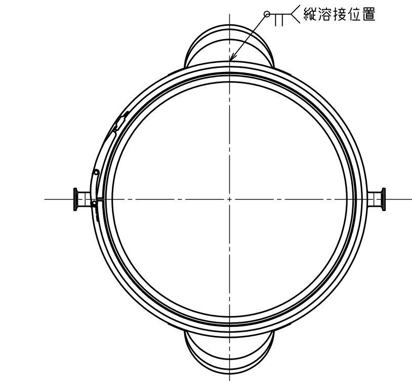
B部詳細図 S = 1 : 1
