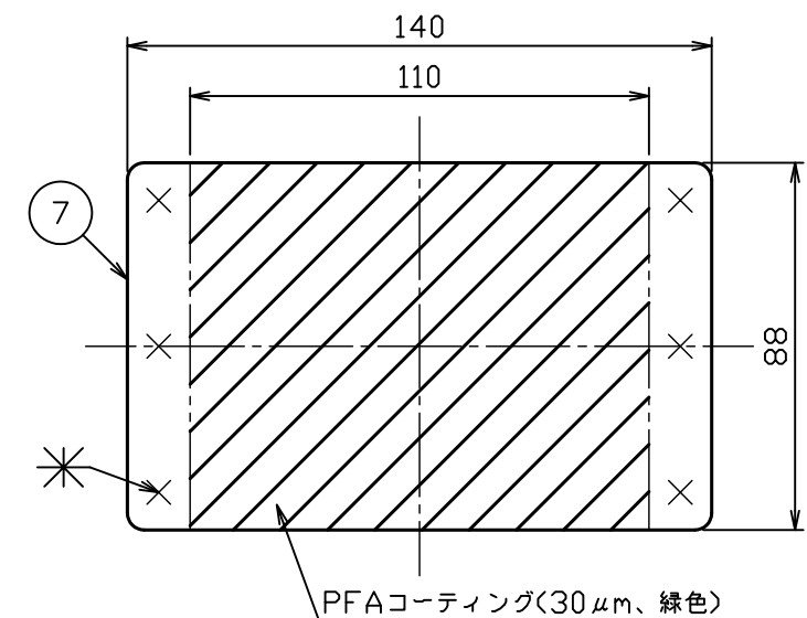
シール座板詳細図 S = 1 : 2
