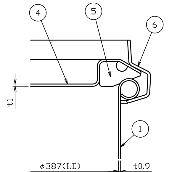
A 部詳細図 S = 1 : 1
