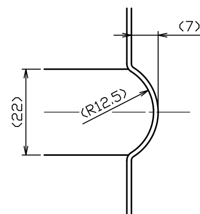
B部詳細図 S = 1 : 1
