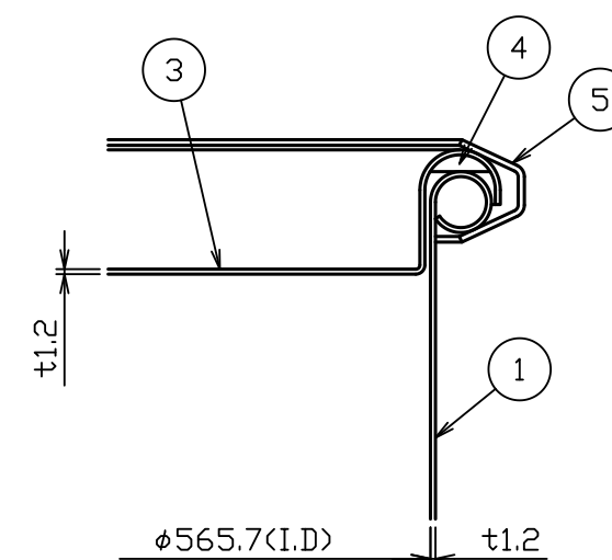
A部詳細図 S = 1 : 2
