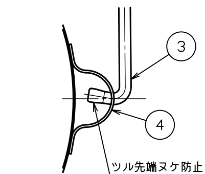
B部詳細図 S = 1 : 2
