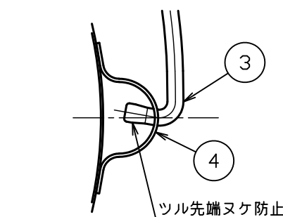
B部詳細図 S = 1 : 2
