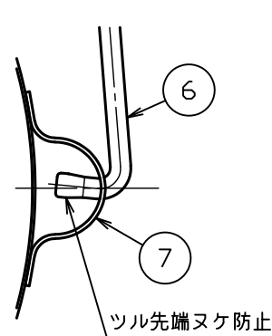
△B部詳細図 S = 1 : 2
