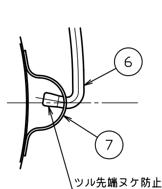
△B部詳細図 S = 1 : 2
