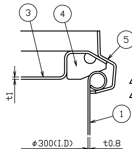
△B部詳細図 S = 1 : 2
