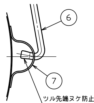
△B部詳細図 S = 1 : 2
